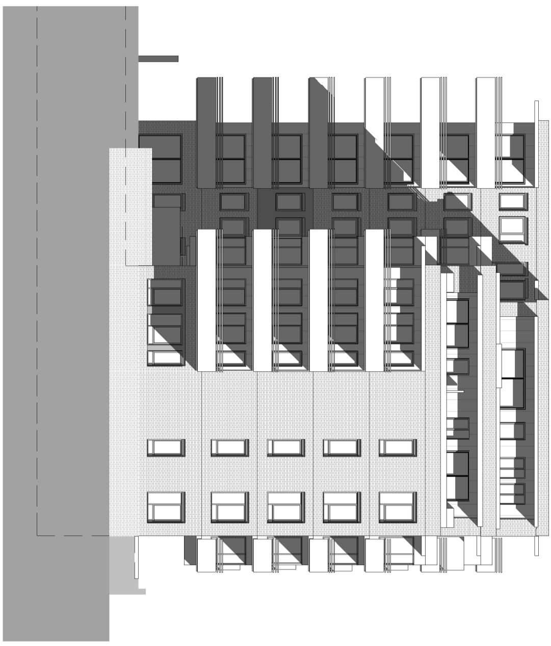
BLOKK B - FASADE SØRVEST - Illustrasjon tegning
